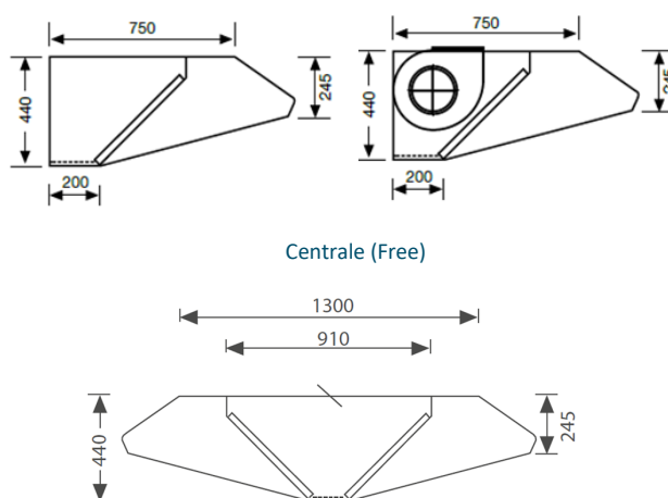
Vue latérale
